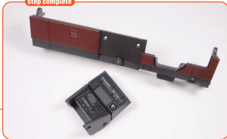
將中央控制台側面板 (R) 53-F 的螺絲孔凹槽和兩個突起部分，對準 53-D 右側的螺絲孔突起和兩個洞孔組裝嵌入，並使用 AP 螺絲 固定。
