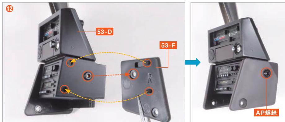
將中央控制台側面板 (R) 53-F 的螺絲孔凹槽和兩個突起部分，對準 53-D 右側的螺絲孔突起和兩個洞孔組裝嵌入，並使用 AP 螺絲 固定。
