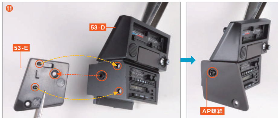
將中央控制台側面板 (L) 53-E 的螺絲孔凹槽和兩個突起部分，對準 53-D 左側的螺絲孔突起和兩個洞孔組裝嵌入，並使用 AP 螺絲 固定。
